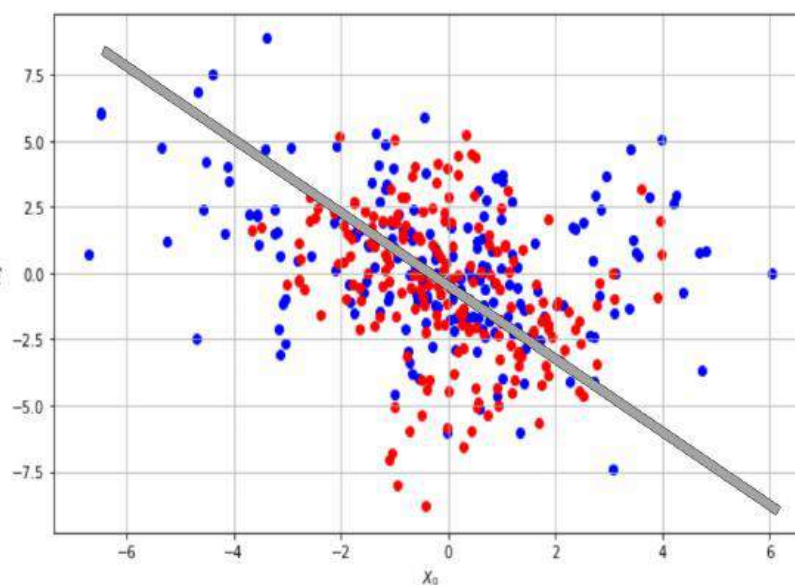
Ilustración 2.5 Regresión lineal con datos no linealmente separables
