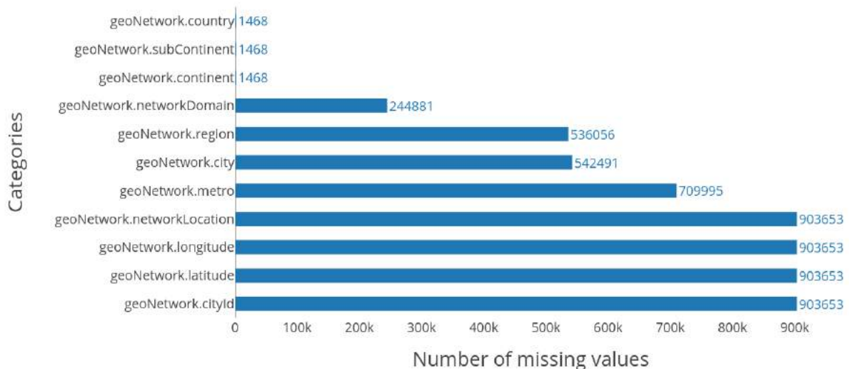
Ilustración 3.5 Valores vacíos en registro geoNetwork
